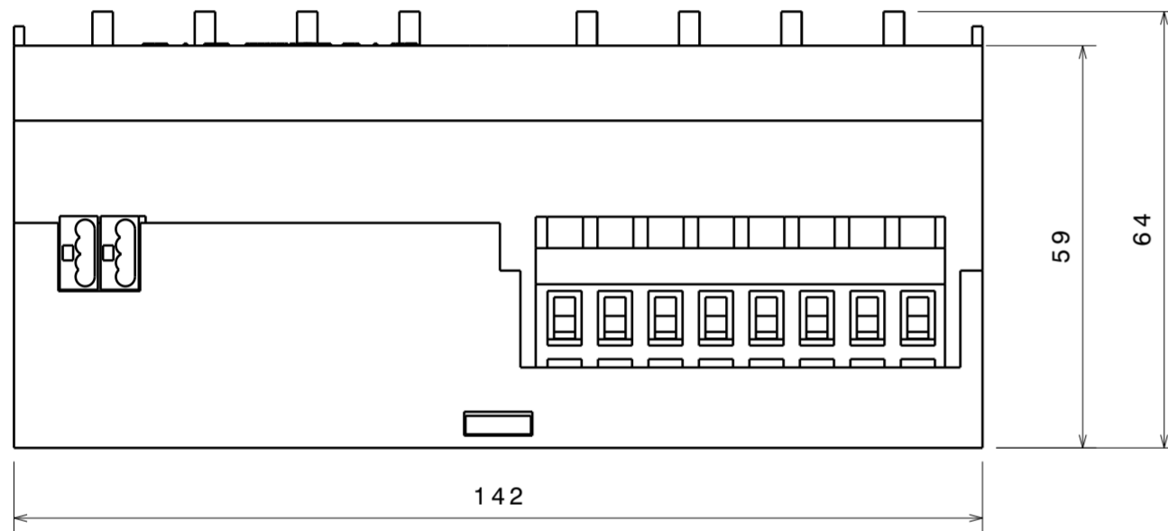
Vista frontale Scala: 1:1
